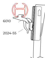
Köpfchen mit Vorsprunggleiter 6010 Breite 15 mm
