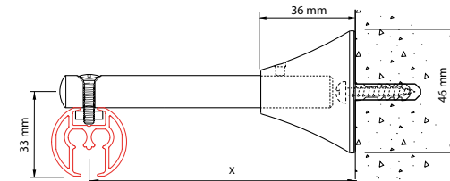
Deckenmontage 5100 mit Deckenträger 5135
