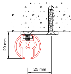
Deckenmontage 5100 mit Deckenträger 5135
