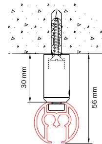
Deckenmontage 5100 mit Deckenträger 4254
