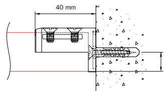
Wandmontage 5100 mit Endträger 5149
