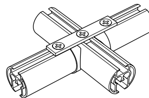
Verbinder 5130
