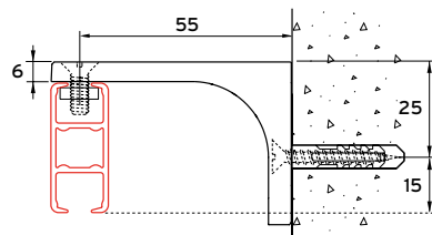
Wandmontage mit Wandträger 4140
