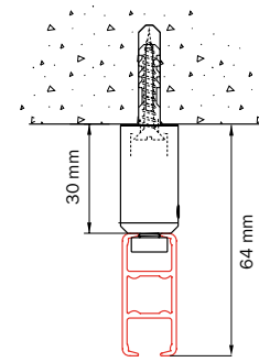
Deckenmontage 4100 mit Lagerträger 4254
