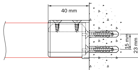
Wandmontage 4100 mit Endträger 4149
