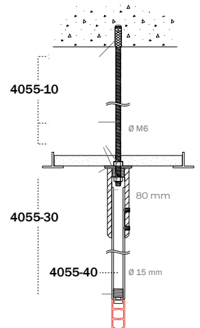
Deckenmontage 4100 an Abhängung 4055-40 mit Montageset 4055-30, Abhängung am Gewindeendset. 4055-10.
