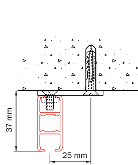
Deckenmontage 4100 mit Deckenabhängiger 4135
